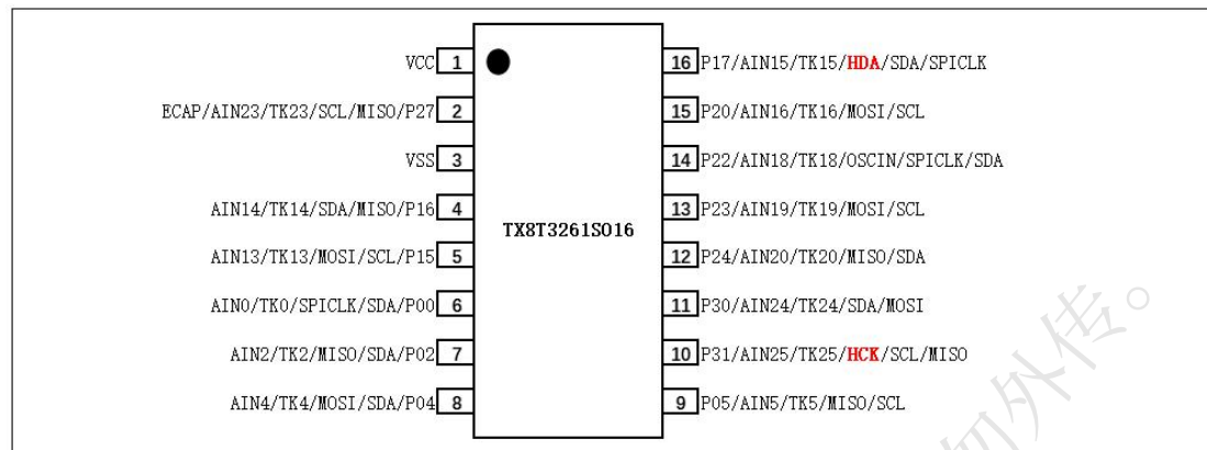
图 1 – TX8T3261S016 (SOP16) 封装图
