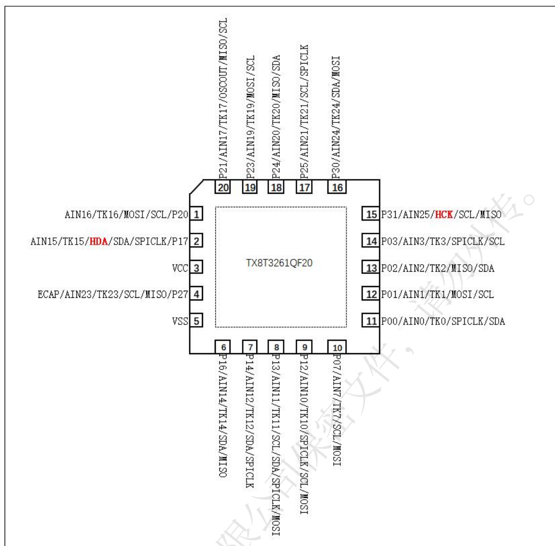
图 5 - TX8T3261QF20 (QFN20) 封装图
