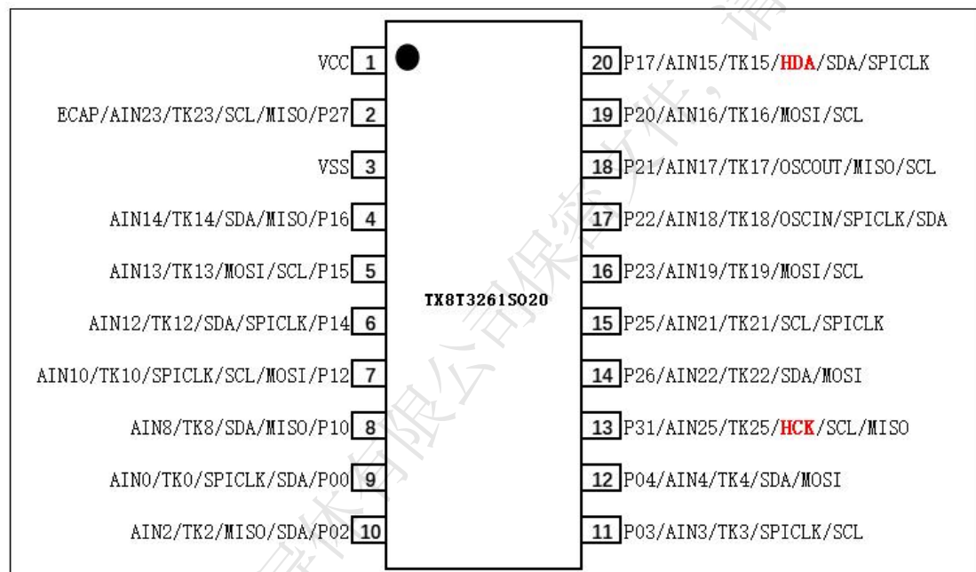
图 2 – TX8T3261S020 (SOP20) 封装图
