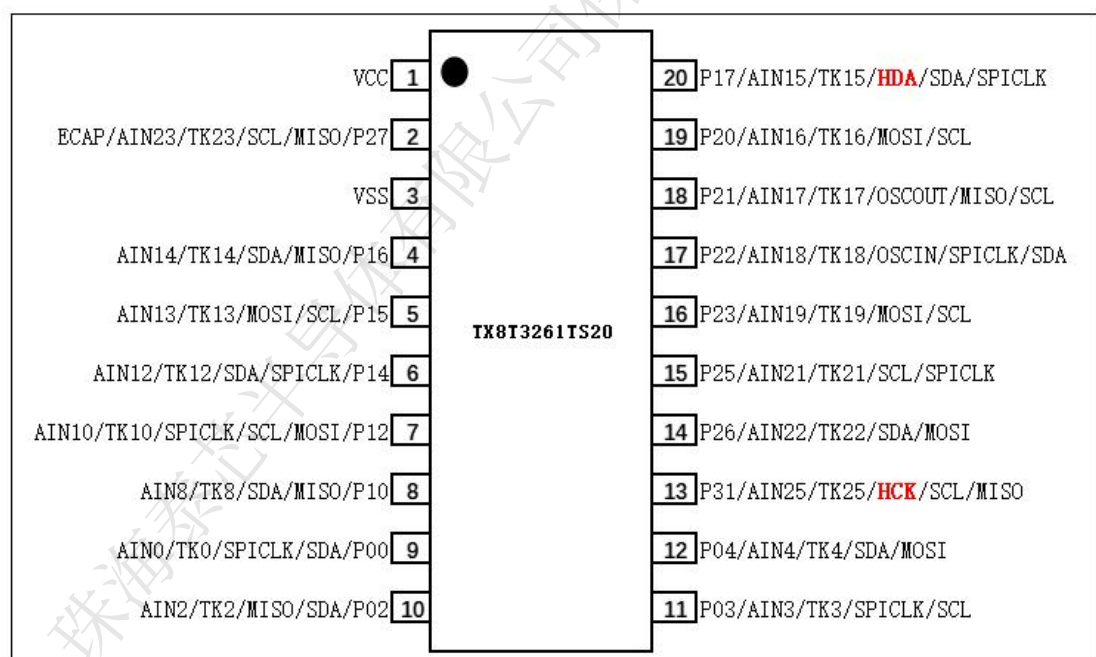
图 4 - TX8T3261TS20 (TSSOP20) 封装图
