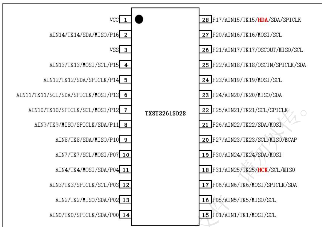
图 3 - TX8T3261S028 (SOP28) 封装图
